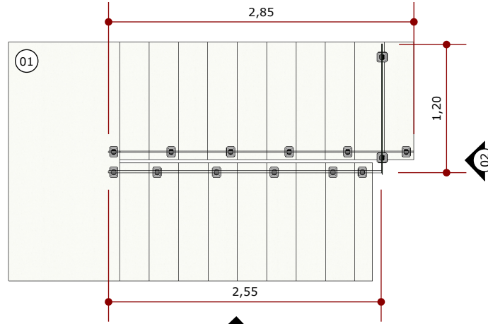
PLANTA BAIXA ESC.: 1/50
