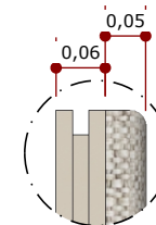
DETALHE LATERAL S/ ESCALA
