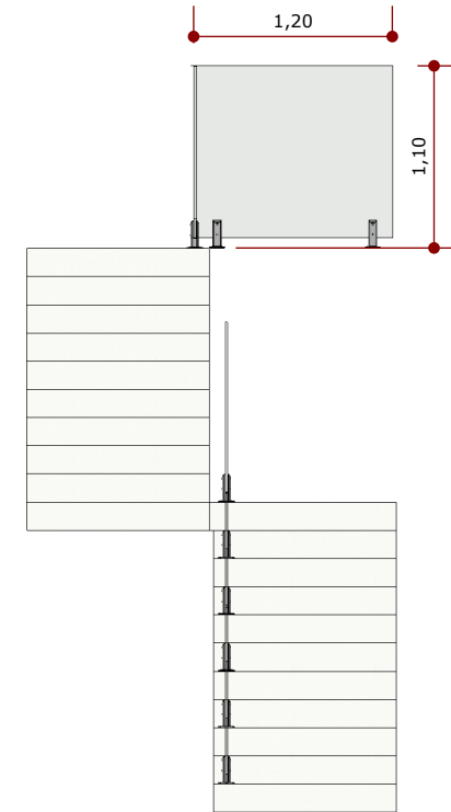
VISTA 02 ESC.: 1/50
