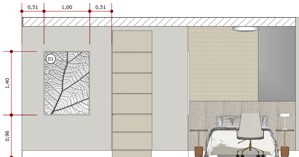
VISTA 08 ESC.: 1/50
