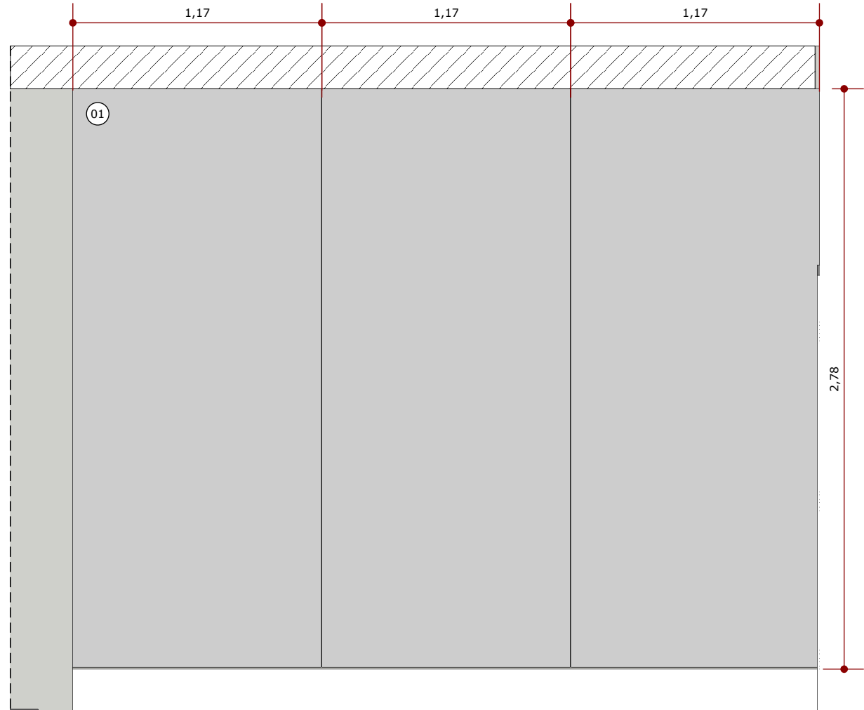
VISTA 01 ESC.: 1/25
