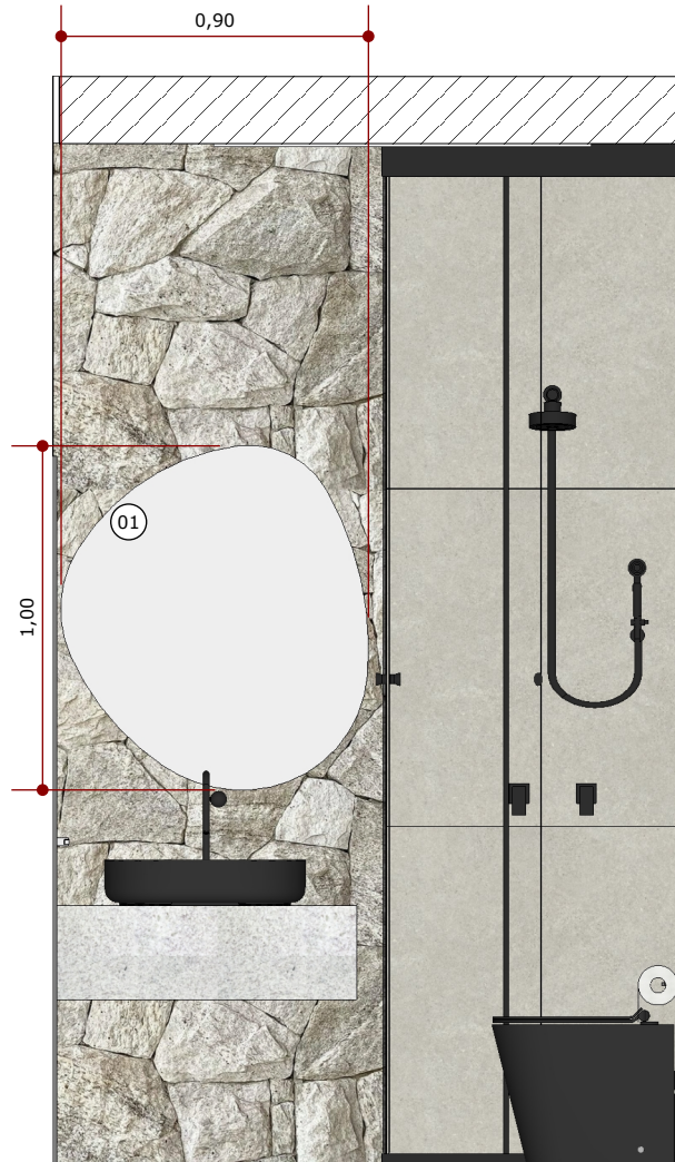
VISTA 01 ESC.: 1/25
