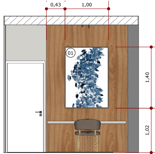
VISTA 12 ESC.: 1/50
