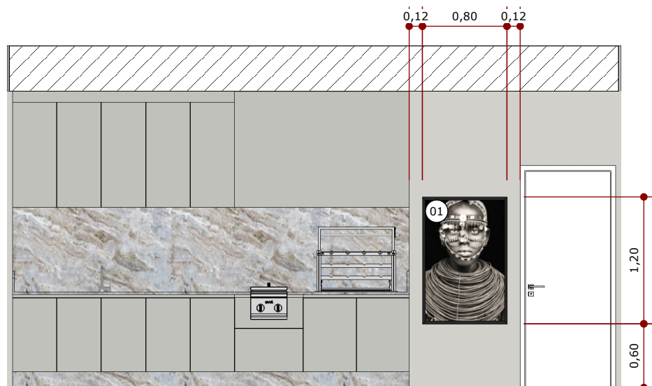
VISTA 03 ESC.: 1/50
