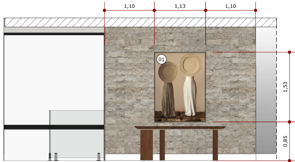
VISTA 06 ESC.: 1/50
