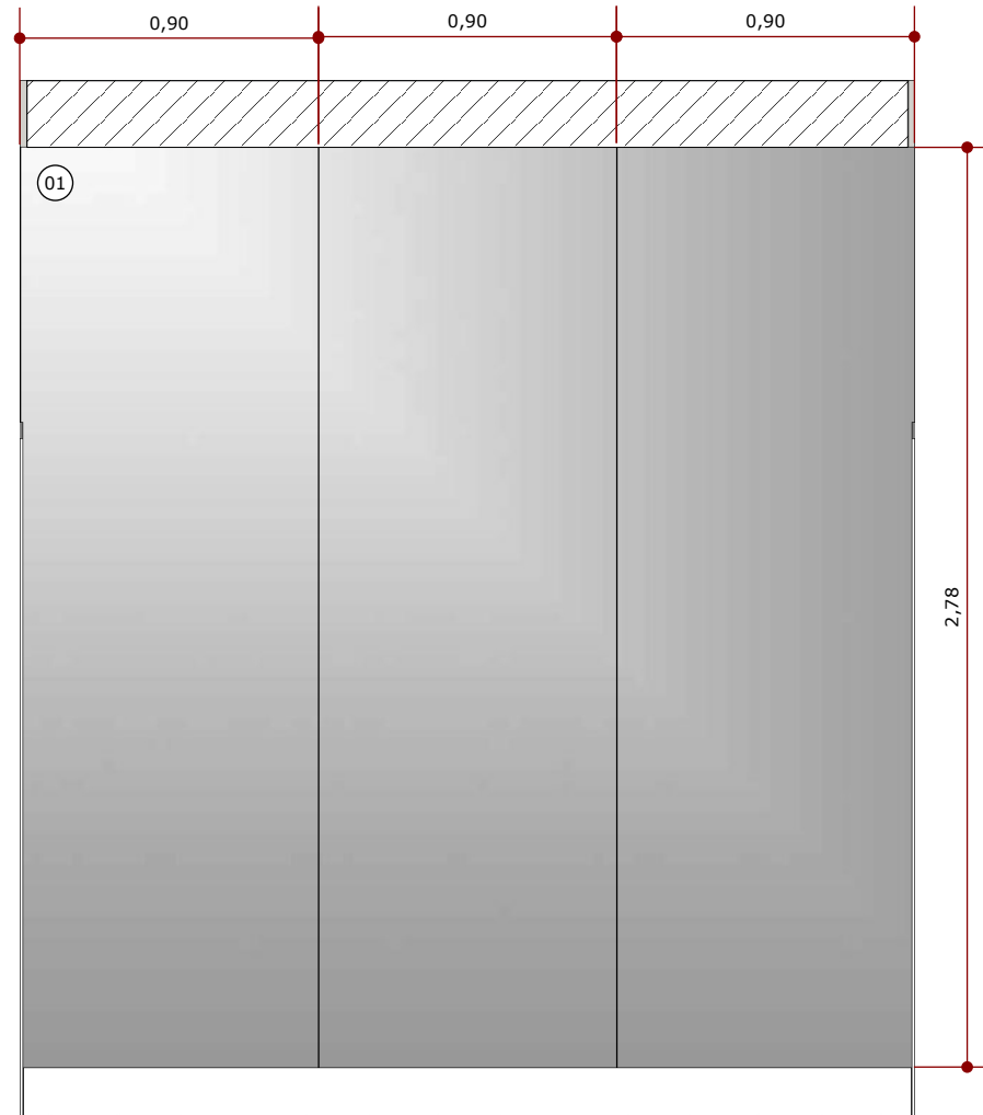
VISTA 01 ESC.: 1/25
