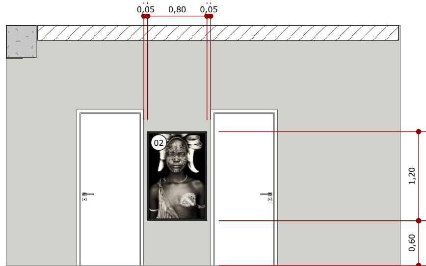
VISTA 02 ESC.: 1/50
