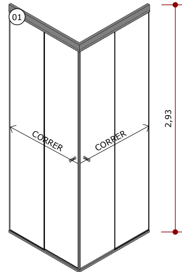
ISOMÉTRICA S/ ESCALA
