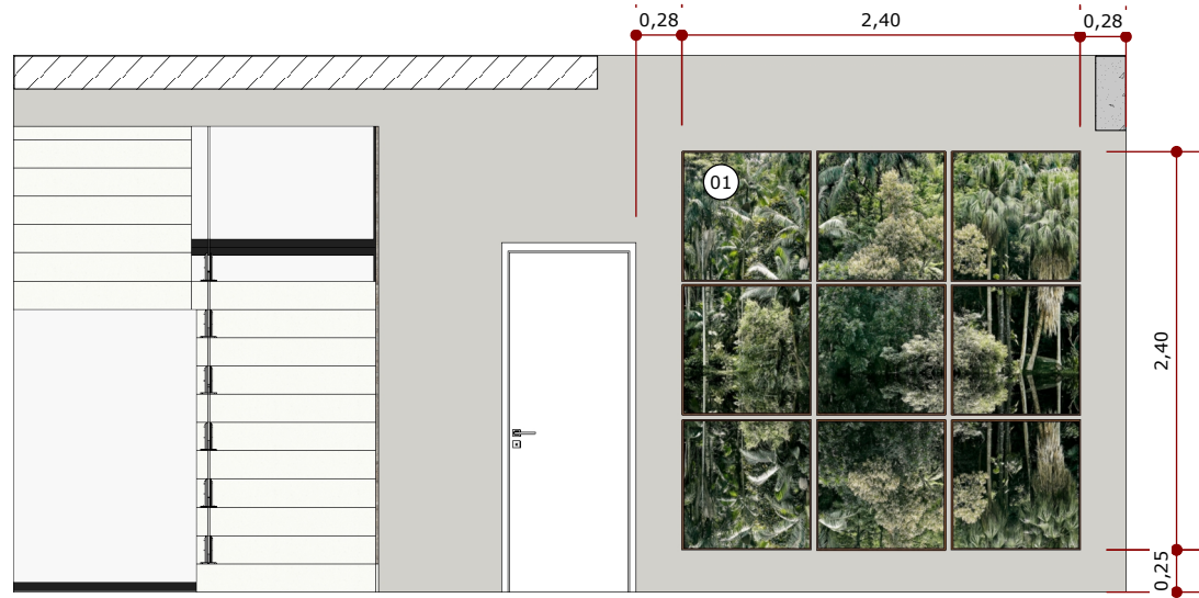
VISTA 01 ESC.: 1/50
