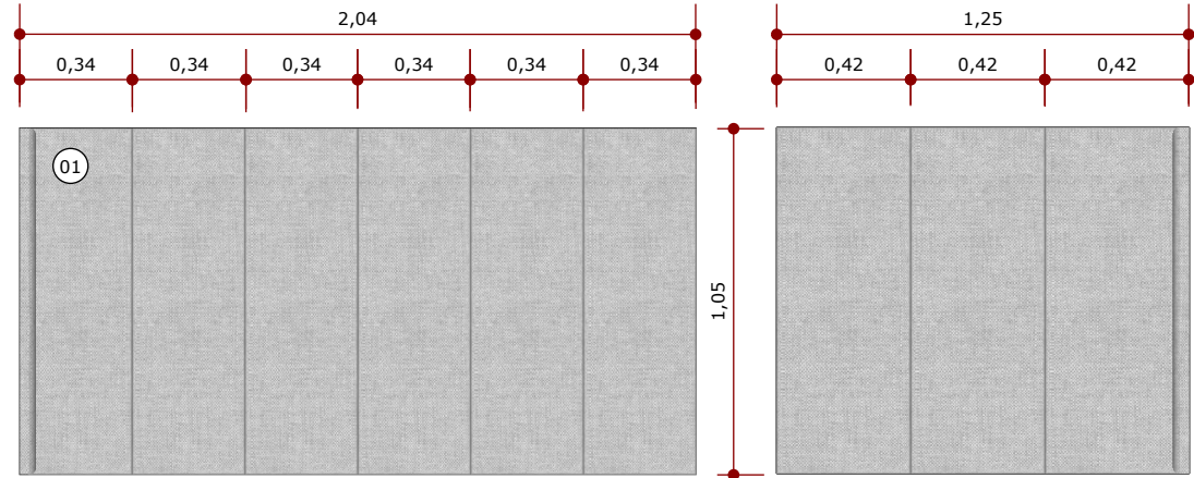
VISTA 01 ESC.: 1/25
