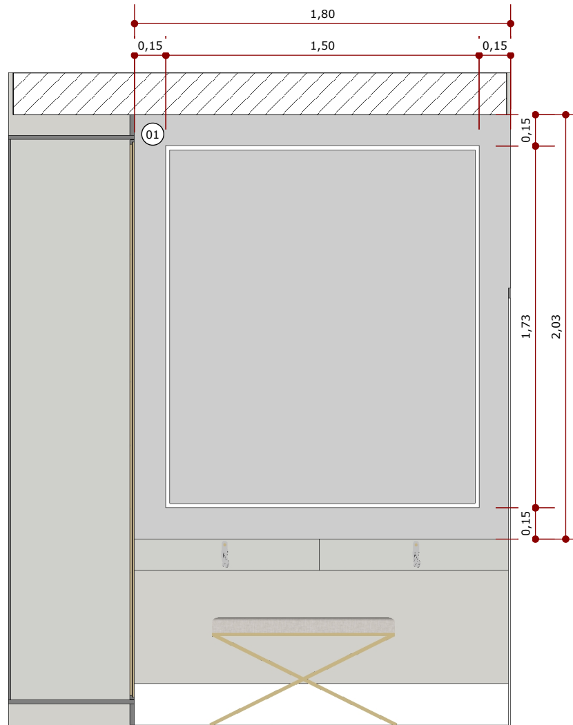
VISTA 01 ESC.: 1/25
