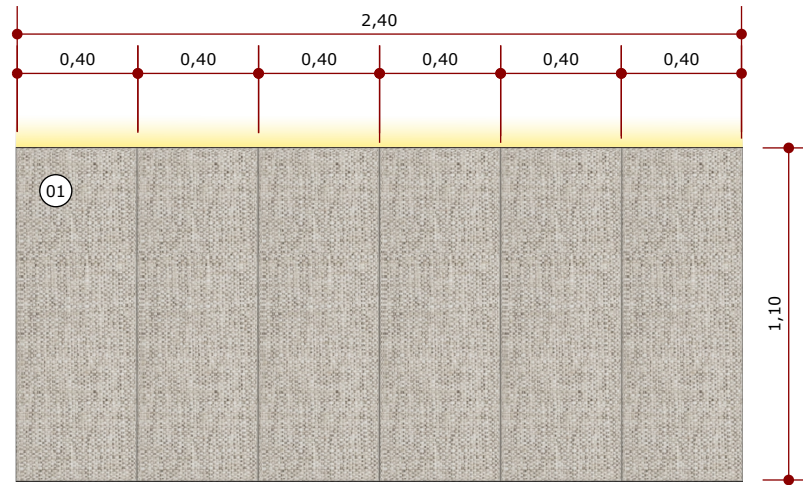
VISTA FRONTAL ESC.: 1/25
