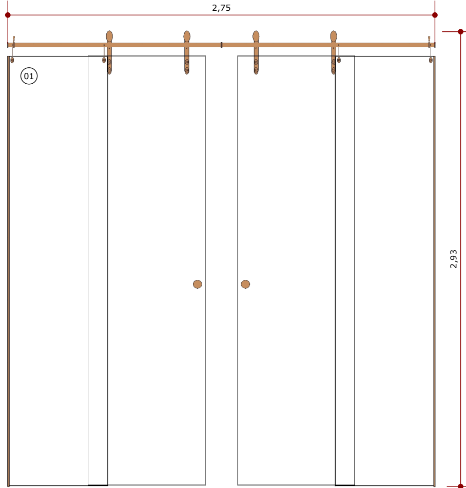
VISTA FRONTAL ESC.: 1/25
