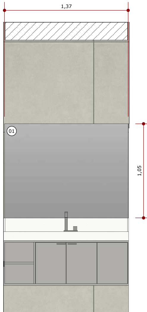
VISTA 01 ESC.: 1/25
