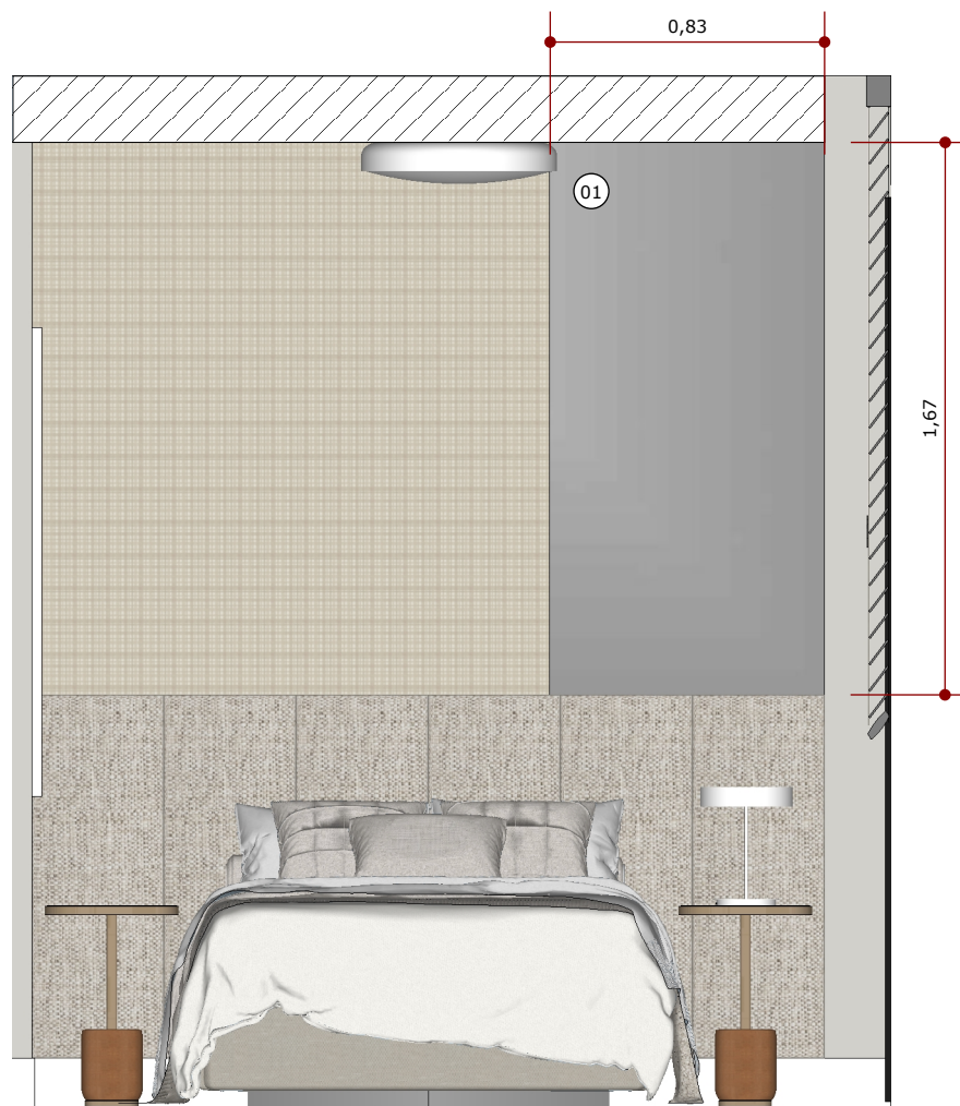
VISTA 01 ESC.: 1/25
