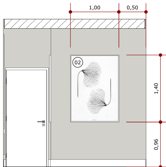
VISTA 09 ESC.: 1/50
