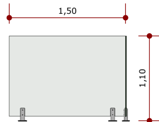
VISTA 02 ESC.: 1/50
