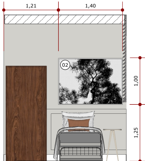
VISTA 05 ESC.: 1/50
