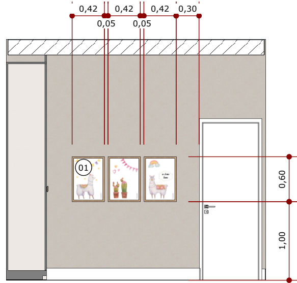
VISTA 10 ESC.: 1/50
