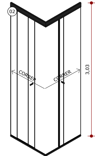
ISOMÉTRICA S/ ESCALA
