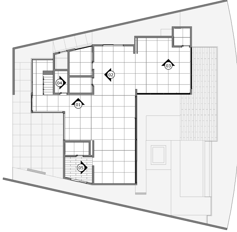
PLANTA GUIA S/ ESCALA
