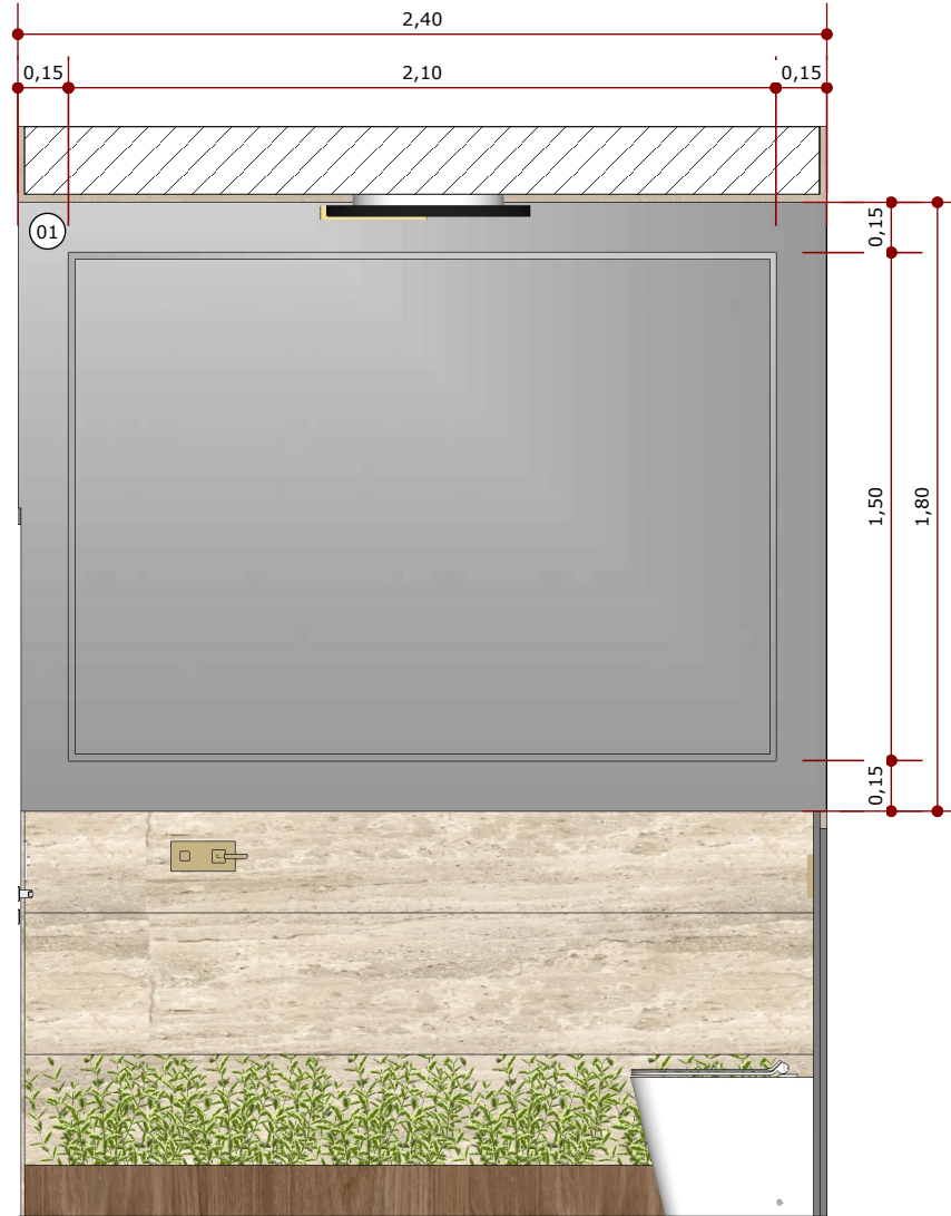
VISTA 01 ESC.: 1/25
