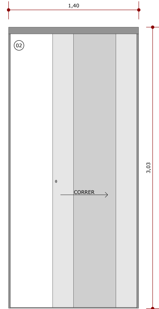
VISTA FRONTAL ESC.: 1/25
