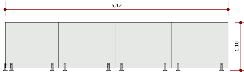
VISTA 01 ESC.: 1/50
